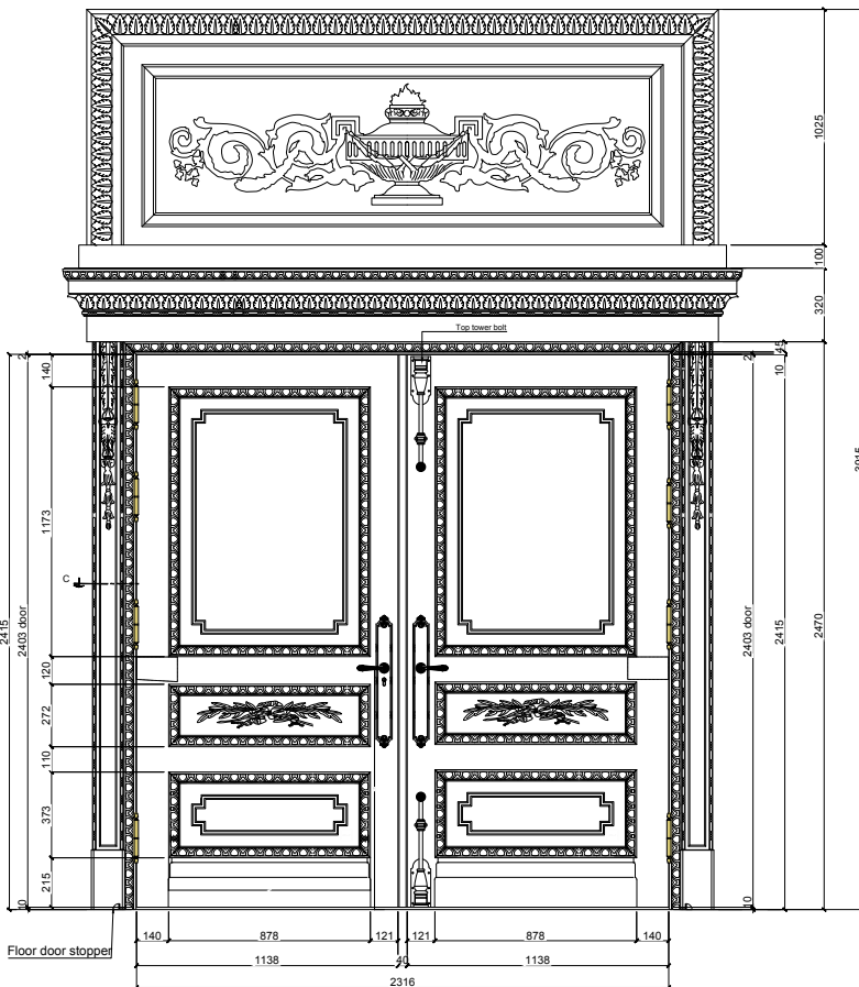
ELEVATION FACE "A" sc.1:10
