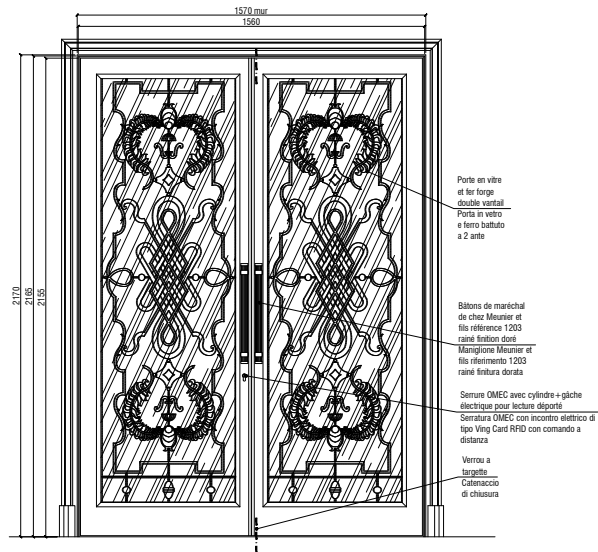
ELEVATION COTE CAVE A VIN - ech. 1:10 PROSPETTO LATO CANTINA - sc. 1:10
