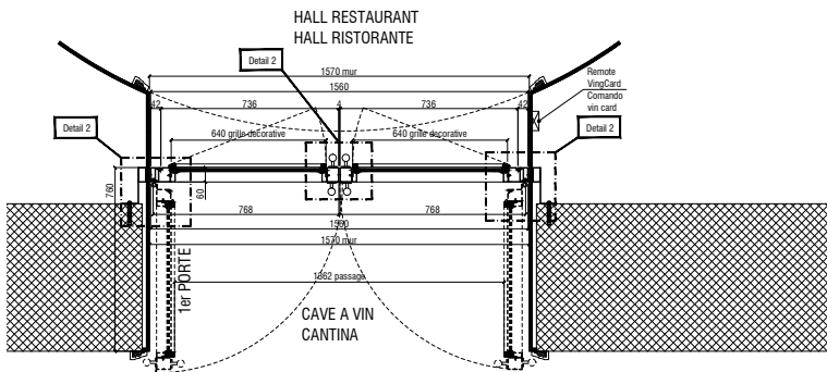
COUPE B-B - ech. 1:10 SEZIONE B-B - sc. 1:10
