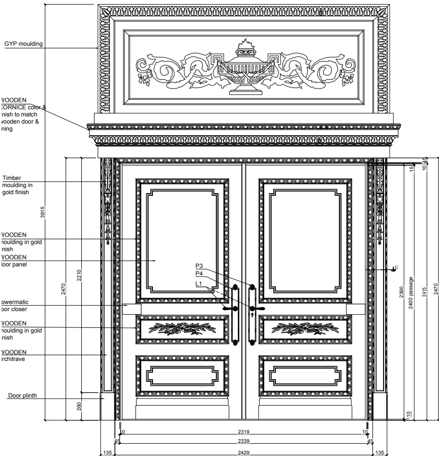
ELEVATION FACE "B" sc.1:10
