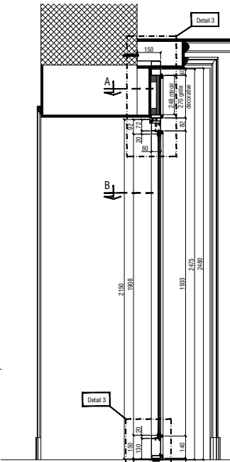
COUPE C-C - ech. 1:10 SEZIONE C-C - sc. 1:10
