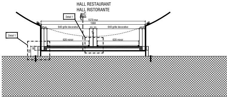
COUPE A-A - ech. 1:10 SEZIONE A-A - sc. 1:10
