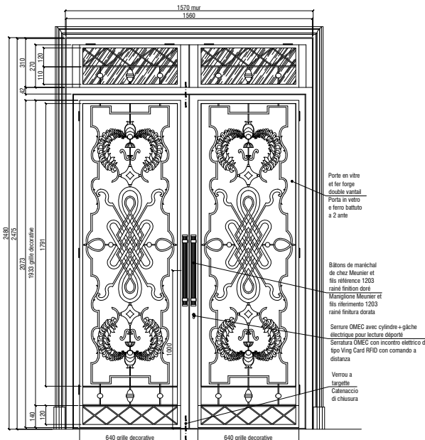
ELEVATION COTE HALL RESTAURANT - ech. 1:10 PROSPETTO LATO HALL DEL RISTORANTE - sc. 1:10
