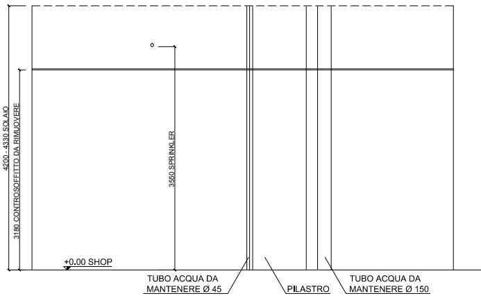
SEZIONE B-B
