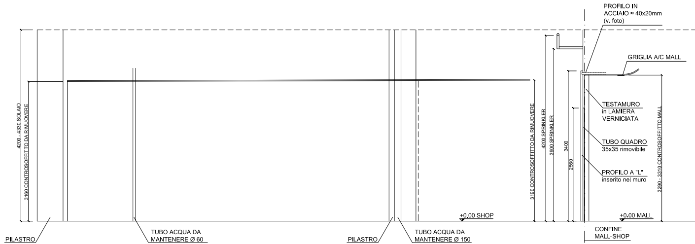
SEZIONE A-A
